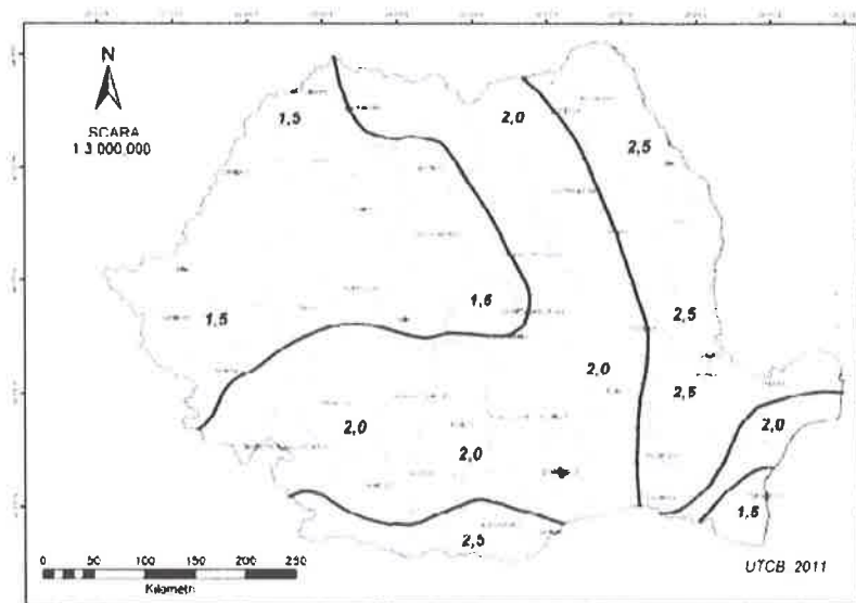
Figura 3.1 Zona valorilor caracteristice ale încărcării din zăpadă pe sol s, kN/m 2 , pentru altitudin A = 1000 m NOTA: Pentru altitudin A = 1000 m valorile s, se determină cu relațiile (3.1) și (3.2)
