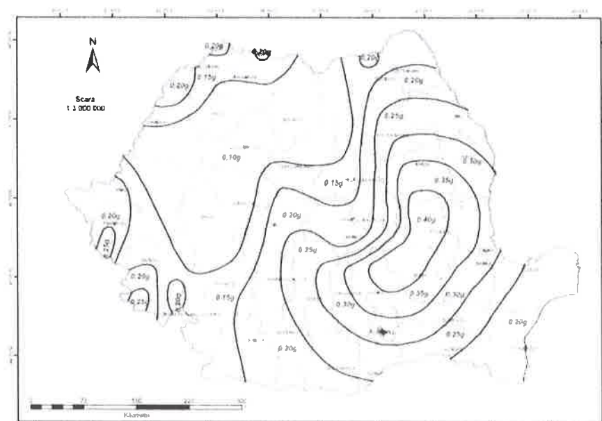
Figura 3.1. România - Zonare valorilor de vârf ale accelerației terenului pentru proiectare pe cu TNR = 225 ani și 20% probabilitate de depășire în 50 de ani
