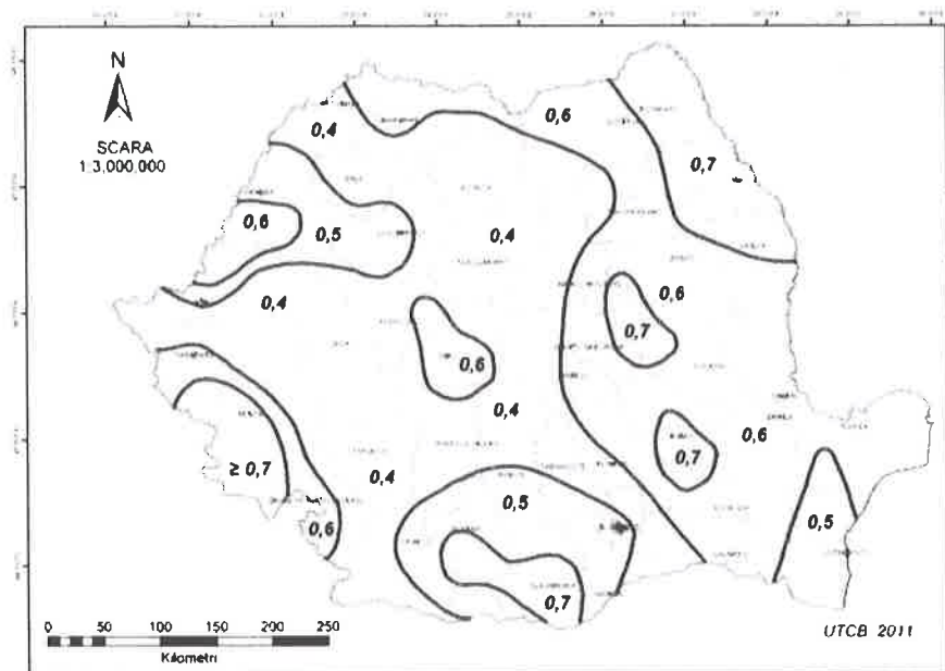
Figura 2.1 Zona valorilor de referință ale presiunii dinamice a vântului, q_s , în kPa, având h_{MR} = 50 m NOTĂ: Pentru altitudini peste 1000m valorile presiunii dinamice a vântului se corectează cu relația (A.3) din Anexa A
