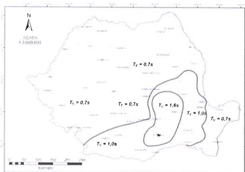
Figura 12. Zonarea terenului Românesc în termeni de perioadă de control (cu T_c ) și spectrul de răspuns
