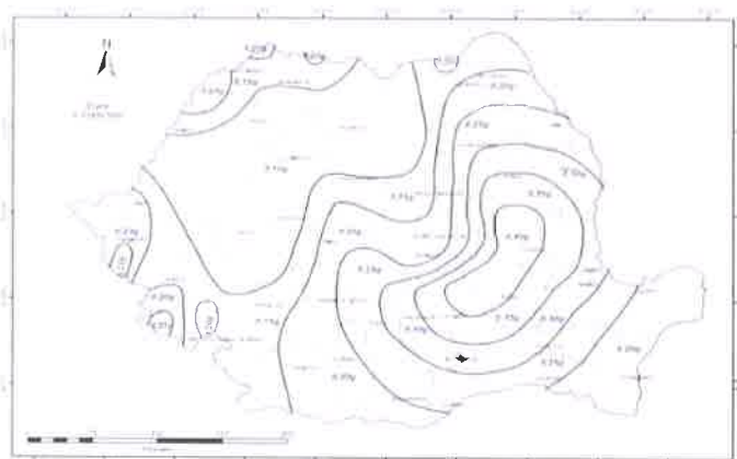
Figura 11. România - Zonarea valorilor de calcul ale nivelului terenului pentru proiectarea cu un T_{RH} = 225 ani și 10% probabilitate de depășire în 50 de ani
